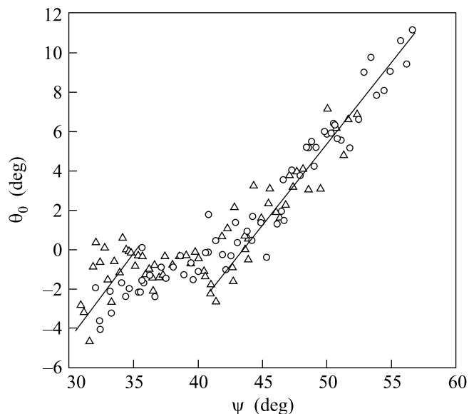
Рис.5. Зависимость угла наклона поверхности в точке касания \theta_0 от угла наклона стенки \psi . Круглые символы относятся к левой стенке, треугольные – к правой
