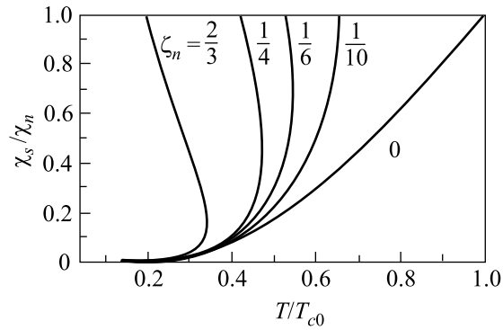
Рис.3. Температурная зависимость спиновой восприимчивости \chi_s(T)/\chi_n при различных значениях параметра \zeta_n
