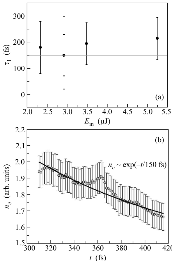
Рис.4 (а) Зависимость времени релаксации носителей заряда в микрообъеме плавленного кварца от энергии возбуждающего импульса. Время релаксации, полученное по нелинейному поглощению ( \Delta ), по третьей гармонике ( \bullet ), по результатам работы [8, 9] (—); (б) зависимость электронной плотности от временной задержки, полученная после преобразований из временного профиля сигнала третьей гармоники
