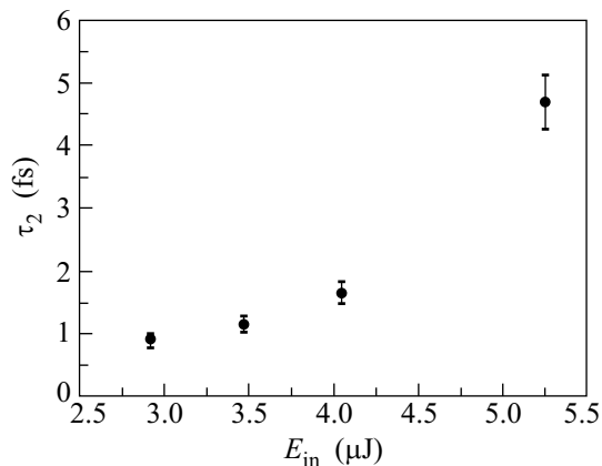
Рис.5. Зависимость времени релаксации нелинейной восприимчивости третьего порядка \chi^{(3)} модифицированного образца плавленного кварца от энергии возбуждающего импульса
