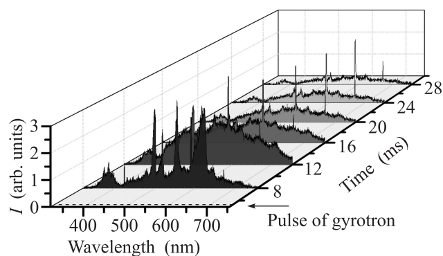
Рис. 3. Динамика спектров, измеренных над поверхностью порошка реголита (смесь #2), спектрометром #2. Интервал между спектрами 4 мс. Импульсное воздействие гиротрона длительностью 2 мс
