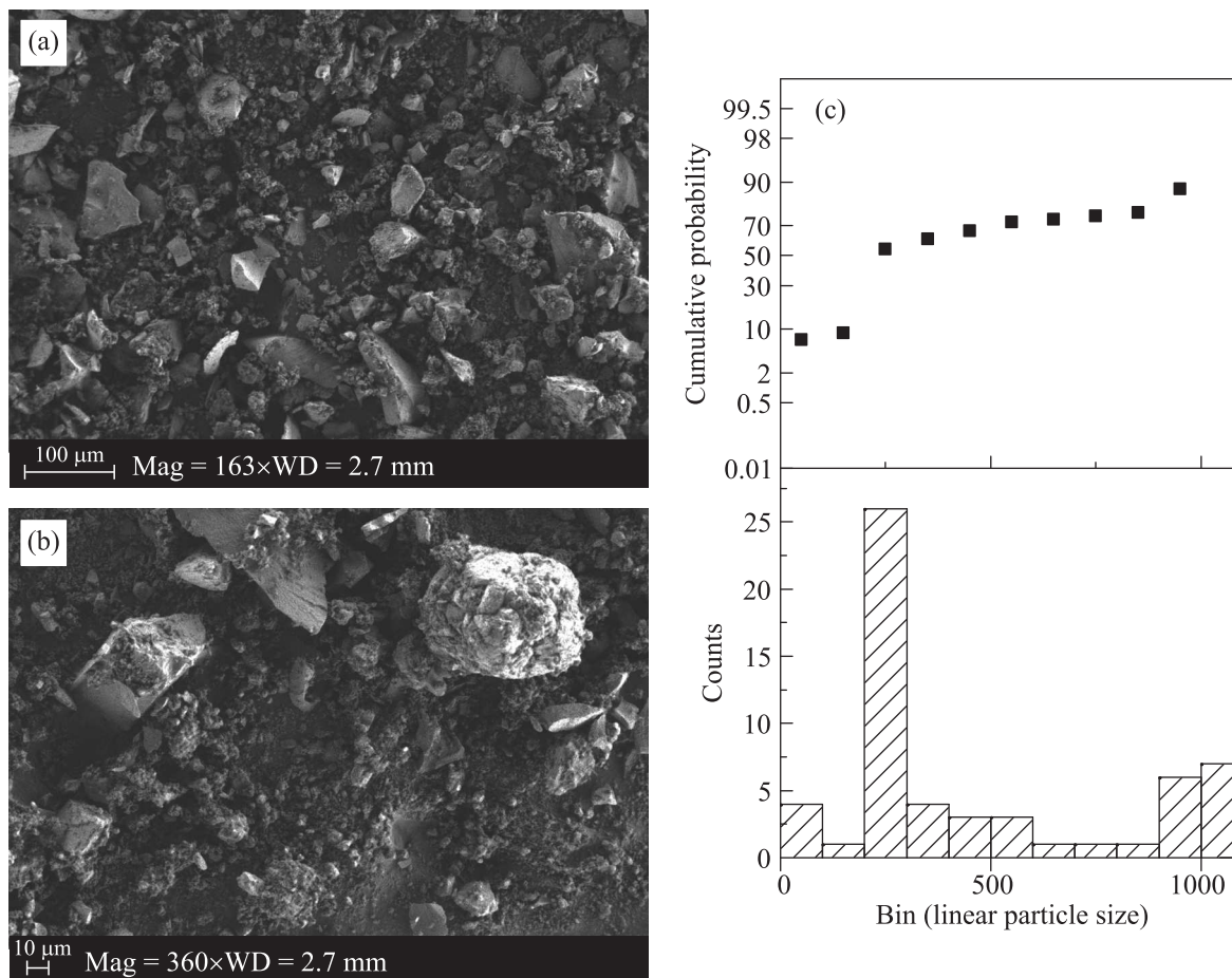
Рис. 2. (а), (b) – Микрофотографии исходного порошка реголита (смесь # 2) в двух масштабах: 100 и 10 мкм. (с) – Для фотографии с масштабом 100 мкм представлены распределения частиц по размерам
