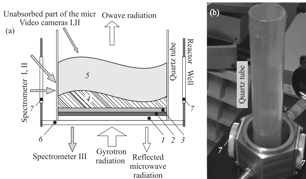
Рис. 1. (а) – Схема эксперимента. 1, 2, 6, 7 – кварцевые пластины; 3 – слой реголита; 4, 5 – плазменный и газовые слои с частицами. Стрелками схематически показаны области приема излучения видеокамерами (I, II) и спектрометрами (I, II, III). (б) – Кварцевая трубка с переопыленным реголитом после воздействия импульса гиротрона. 7 – Диагностические патрубки с кварцевыми пластинами. Реголит (смесь # 2). Атмосфера. Энергия СВЧ импульса 0.07 \text{ кДж} \cdot \text{см}^{-2} . Длительность СВЧ 1.5 мс
