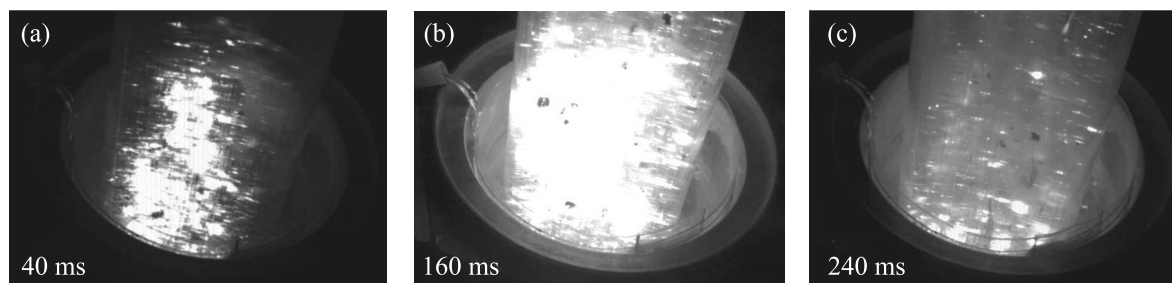
Рис. 4. Видеокадры эволюции во времени ансамбля частиц реголита (смесь # 2) в реакторе. Импульсное воздействие гиротрона длительностью 2 мс. На фотографиях указано время после окончания СВЧ импульса гиротрона. Выдержка 0.2 мс
