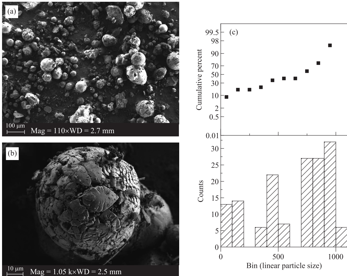
Рис. 5. (а), (b) – Микрофотографии осажденного на стенки реактора порошка реголита (смесь # 2) в двух масштабах: 100 и 10 мкм. (с) – Для фотографии с масштабом 100 мкм представлены распределения частиц по размерам
